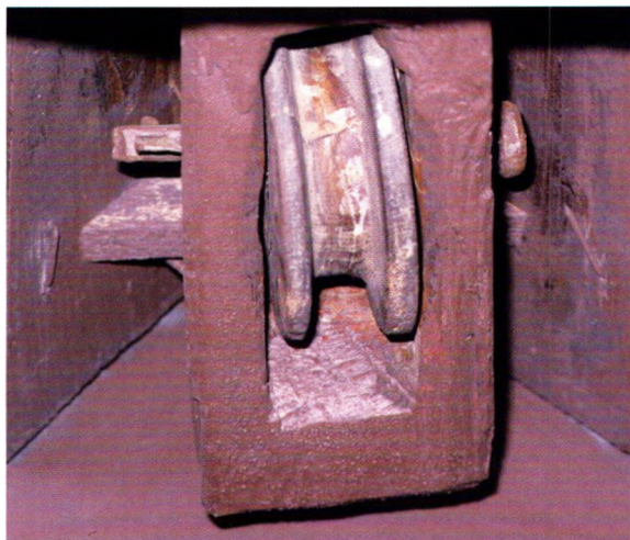
Abb. 22 Die Rolle für den Lastenaufzug im Dachgeschoss
